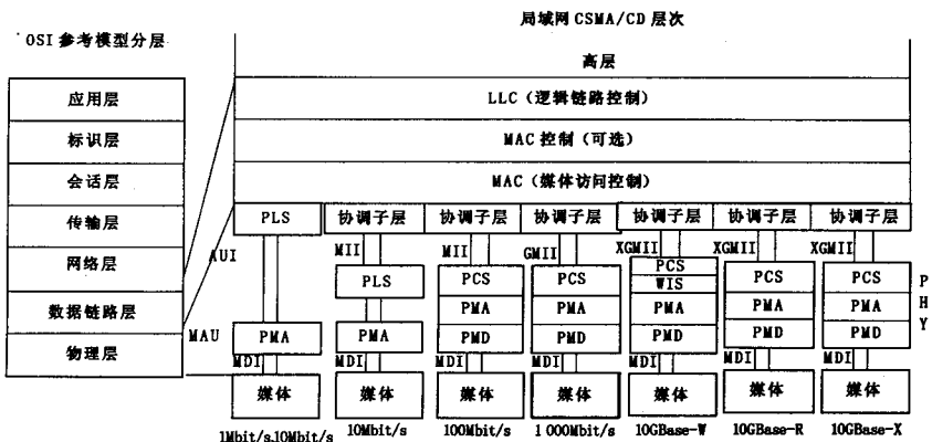
图 1 以太网接口分层
